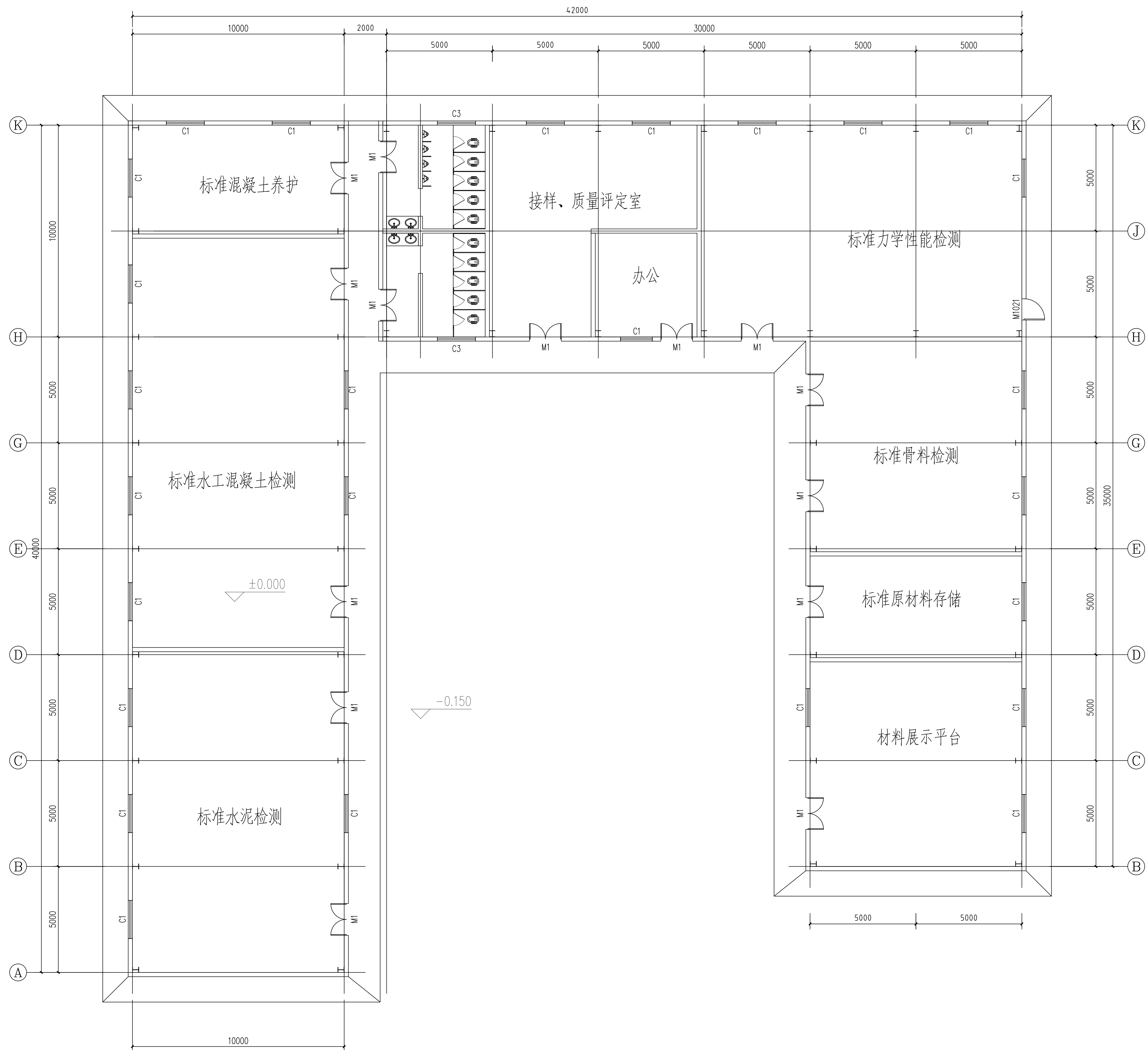
材料检测实训场平面布置图
