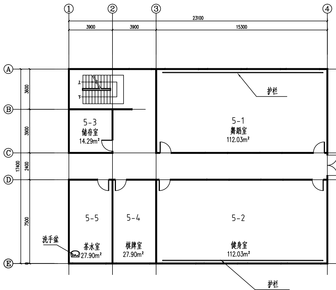
水电实训楼五层平面图
